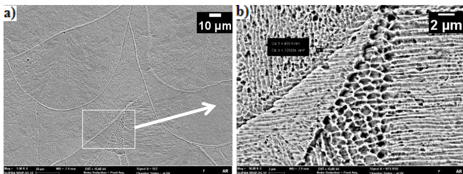
Figura 40 – Morfologia da estrutura de solidificação entre os filetes. Amostra fabricada FSL. FESEM: a) 1.500x, b) 10.000x – Nital 7%.
