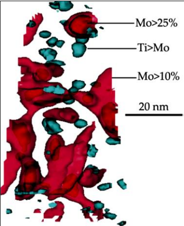
Figura 16 – Geometria dos precipitados gerada a partir das informações obtidas por APT nas fatias analisadas (conforme mostrado na figura 15). Fonte: Jägler et al (2014)
