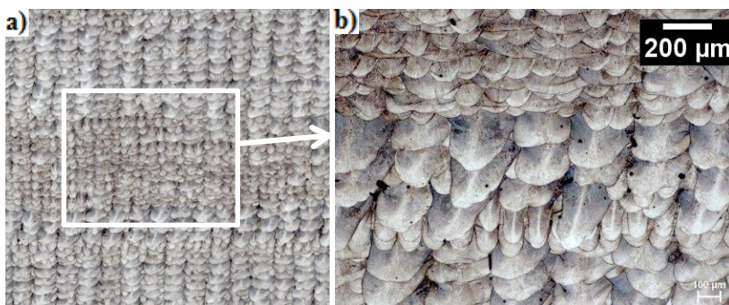
Figura 37 – Filetes da amostra como-fabricada FSL, polida e atacada, observados com duas ampliações: a) aprox. 25X b) aprox. 50x – Nital 7%.
