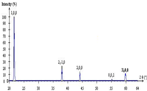
Figura 116 - Difratoograma simulado em software CaRIne da fase S A8B .
