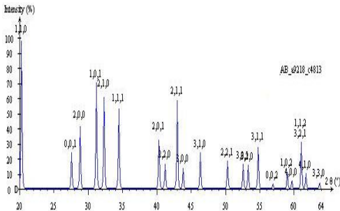
Figura 119 - Difratoograma simulado em software CaRIne da fase FeMo-AB.
