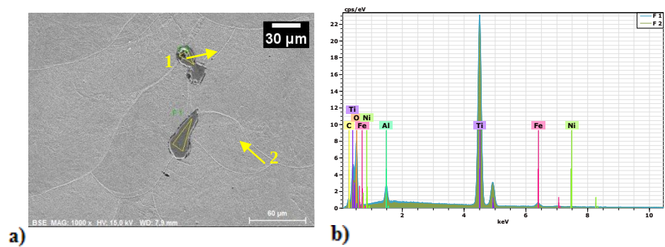
Figura 45 – Amostra como-fabricada: a) Inclusões não metálicas localizadas nos contornos dos filetes da amostra como-fabricada FSL, observada a 1000X com elétrons secundários; b) Espectro de energia dispersiva de raios-X.
