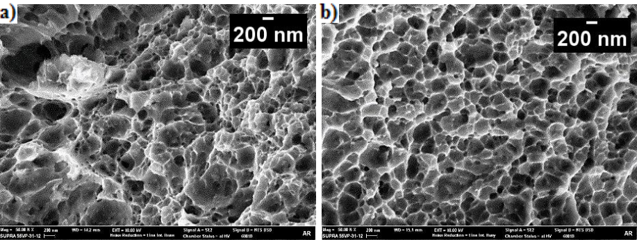
Figura 112 – Superfície de fratura do CP 600_10 - FESEM a aprox. 50kX: a) centro, b) lateral.
