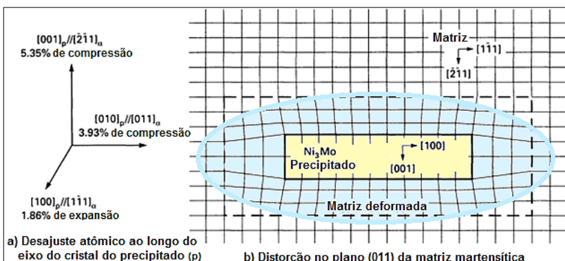
Figura 14 – Diagrama mostrando (a) tensões provocadas pelo desajuste atômico do precipitado de \text{Ni}_3\text{Mo} , e (b) distorções causadas pelo precipitado \text{Ni}_3\text{Mo} na matriz martensítica. Fonte: Shimizu e Okamoto, 1971 apud ASM HANDBOOK, 1991 (Adaptado)
