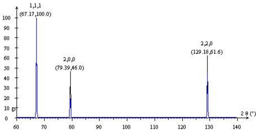
Figura 80 - Difratoograma simulado em software CaRIne da fase CFC.
