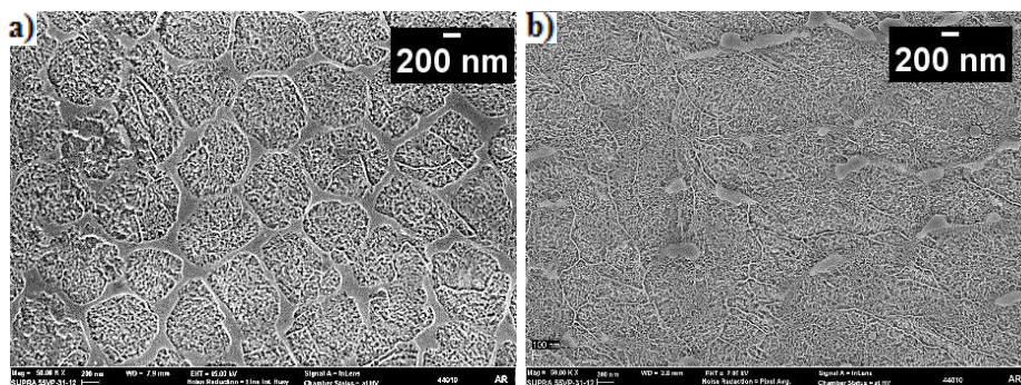
Figura 48 – Microestrutura da amostra 440_10. FESEM: a-b) 50.000X - Ataque Nital 7%.
