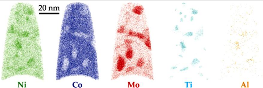
Figura 15 – Concentrações dos principais átomos de soluto nos precipitados formados em um aço maraging envelhecido, avaliadas através de APT em uma amostra de 10 nm de espessura. Fonte: Jägler et al (2014).
