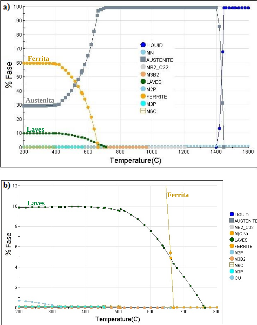
Figura 22 – a) Diagrama de fases multicomponentes da liga Maraging C300 obtido através do software JMatPro . b) Visualização da faixa de temperatura de 200 a 800 °C, com fases presentes em baixo percentual (até 12%). Fonte: Autor.
