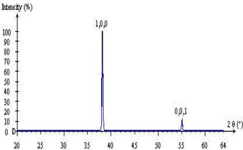
Figura 114 - Difratoograma simulado em software CaRIne da fase \omega .
