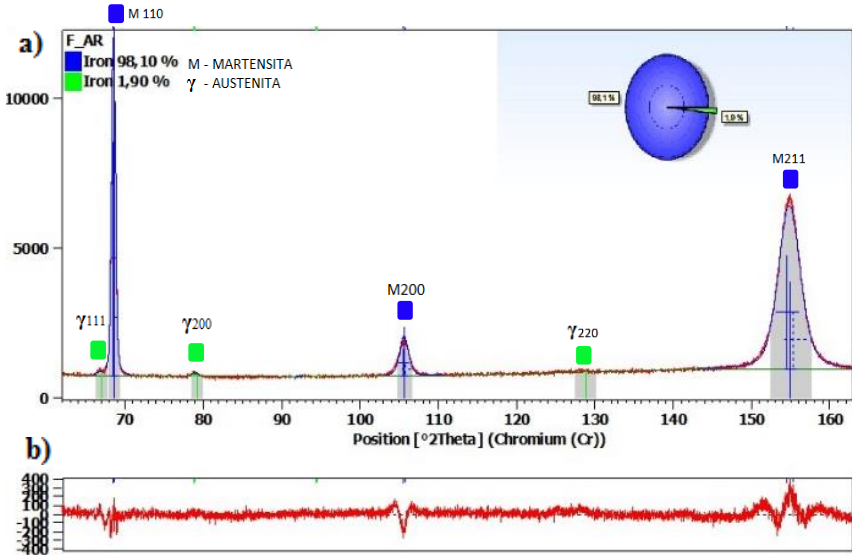
Figura 74 - a) Difractograma da amostra fabricada FSL, com quantificação de fase via Rietveld , b) Gráfico de diferença entre medida e ajuste da curva da quantificação.
