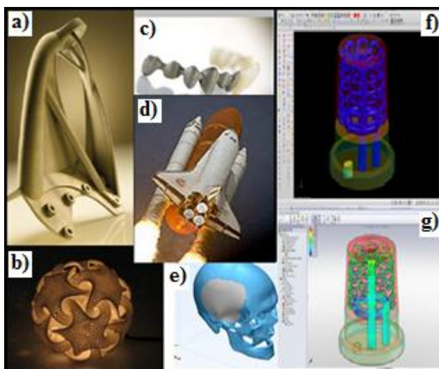
Figura 02 – Exemplos de produtos fabricados por FSL. a) Suporte estrutural; b) escultura metálica; c) prótese dentária; d) componentes aeroespaciais; e) prótese craniana; f-g) inserts com canais para refrigeração de moldes. Adaptada de Concept Laser (2011).
