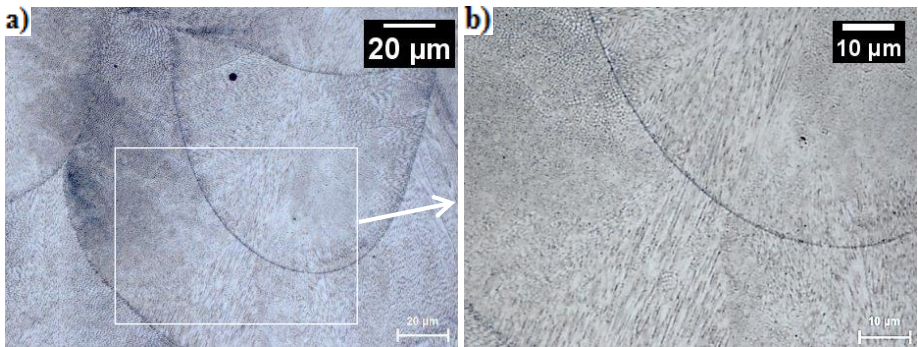
Figura 39 – Orientação de crescimento da estrutura entre os filetes. Amostra fabricada FSL. Microscopia Óptica: a) 500x, b) 1.000x – Nital 7%.
