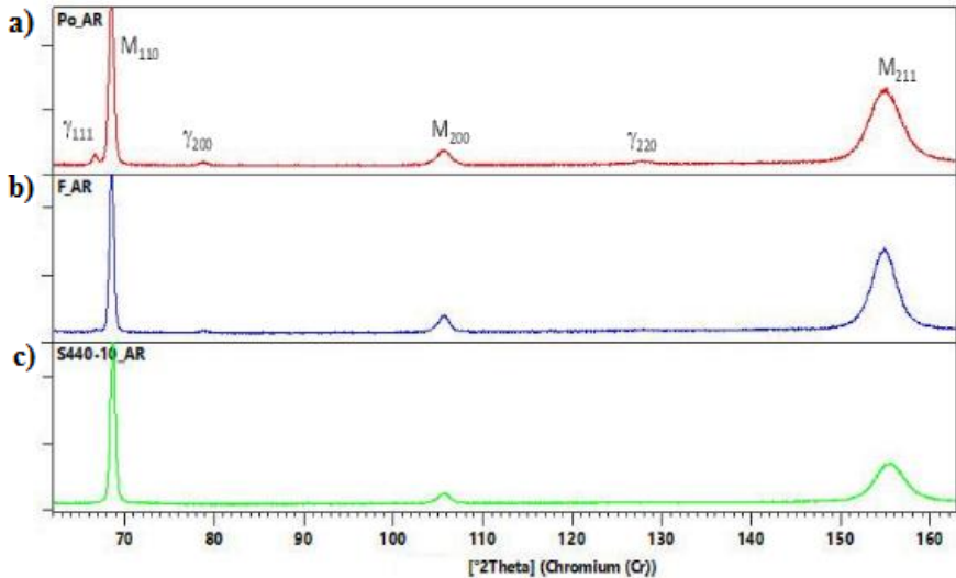
Figura 72 - Comparativo dos difratograma obtidos com a fonte de Cromo. a) pó metálico, b) material fabricado FSL, c) solubilizado à 817°C / 1h, seguido de envelhecimento a 440_10 h.
