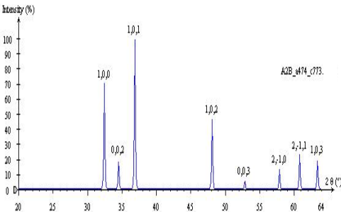
Figura 120 - Difratograma simulado em software CaRline da fase Fe 2 Mo 2 A 2 B .
