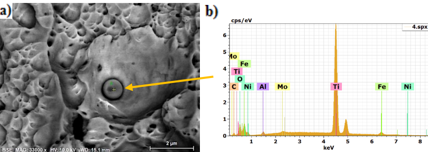
Figura 90 – a) imagem FESEM em aprox. 33.000X; b) Espectro de EDS da partícula. Tabela 28 – Composição química da partícula indicada na Figura 86, obtida através de EDS.
