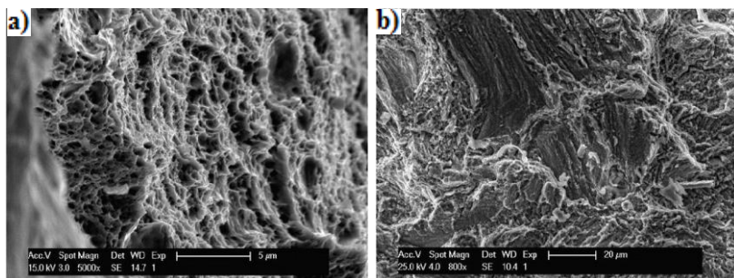
Figura 20 – (a) Amostra fabricada com formação de dimples e fratura dúctil. (b) Amostra envelhecida com fratura frágil do tipo inter e transgranular. Fonte: Kempen et al (2011)
