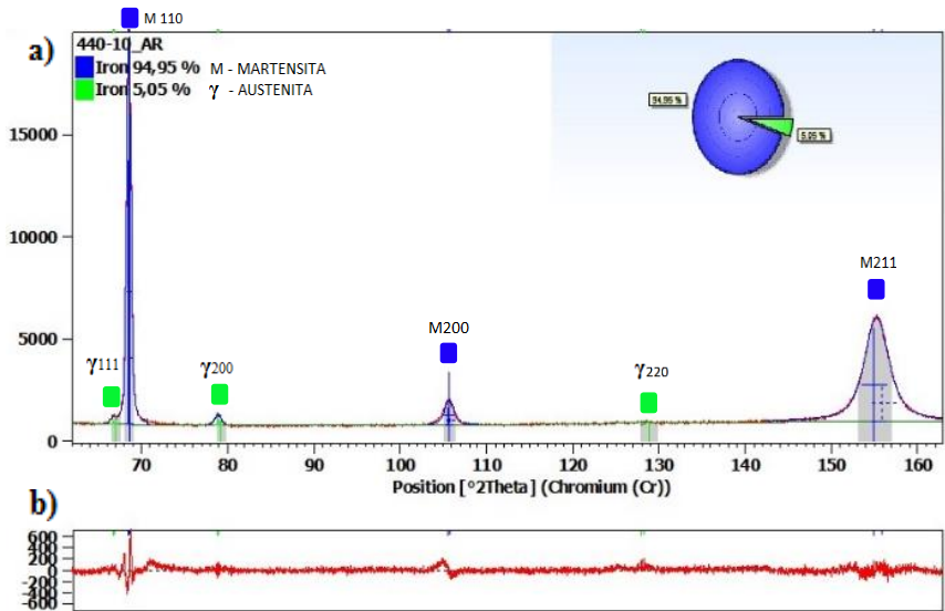
Figura 76 - a) Difractograma com quantificação de fase via Rietveld da amostra envelhecida a 440 °C durante 10h, b) Gráfico de diferença entre medida e ajuste da curva da quantificação.
