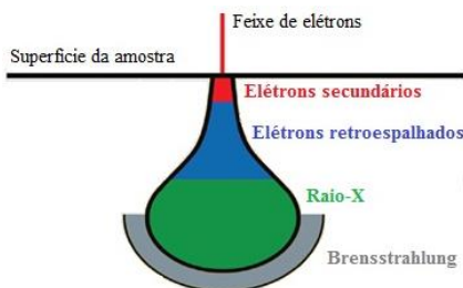
Figura 61 – Ilustração esquemática da interação do feixe de elétrons com a amostra. Fonte: Bruker, (2011).
