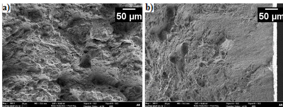
Figura 97 – Superfície de fratura do CP 4805, FESEM aprox. 500X: a) centro, b) lateral.
