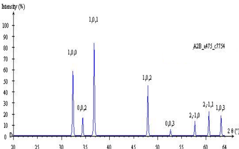
Figura 121 - Difratograma simulado em software CaRline da fase Fe 2 Mo 2 A 2 B
