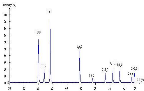
Figura 124 - Difratograma simulado em software CaRIne da fase Ni 3 (Ti, Mo) 2 A 8 B .
