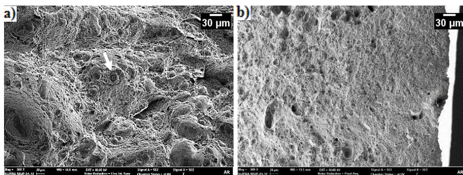
Figura 86 – Superfície de fratura do CP observada em aprox. 500X: a) centro, b) lateral.
