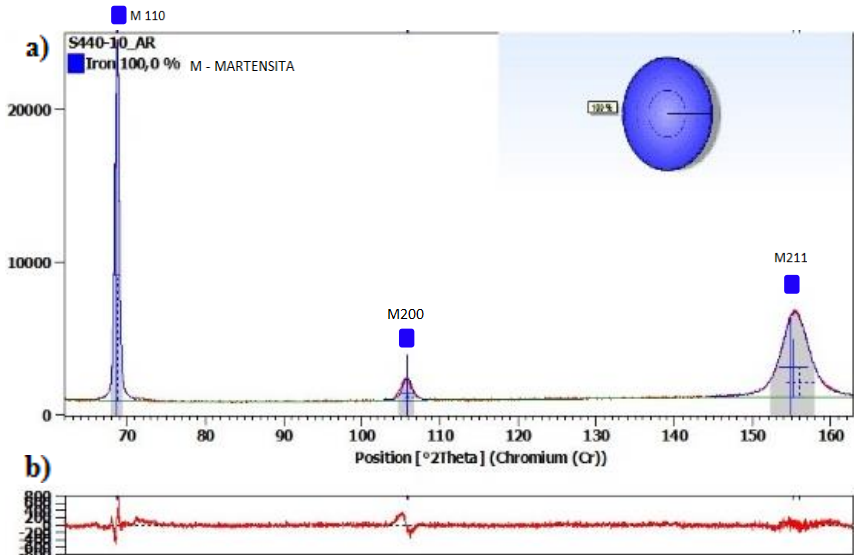
Figura 75- a) Difractograma com quantificação de fase via Rietveld , da amostra solubilizada a 817 °C/1h, envelhecida a 440 °C durante 10h, b) Gráfico de diferença entre medida e ajuste da curva da quantificação.
