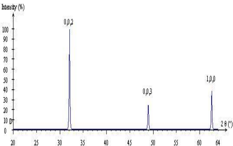
Figura 115 - Difratoograma simulado em software CaRIne da fase \chi_{A_3B} .
