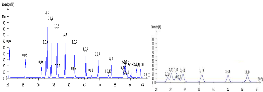
Figura 118 - Difratoograma simulado em software CaRIne da fase \mu_h -A 7 B 6 .
