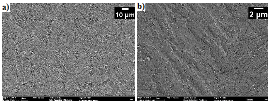
Figura 52 – Microestrutura da amostra S_440_10 atacada com Nital 7%. FESEM: a) 1.500X, b) 10.000X.
