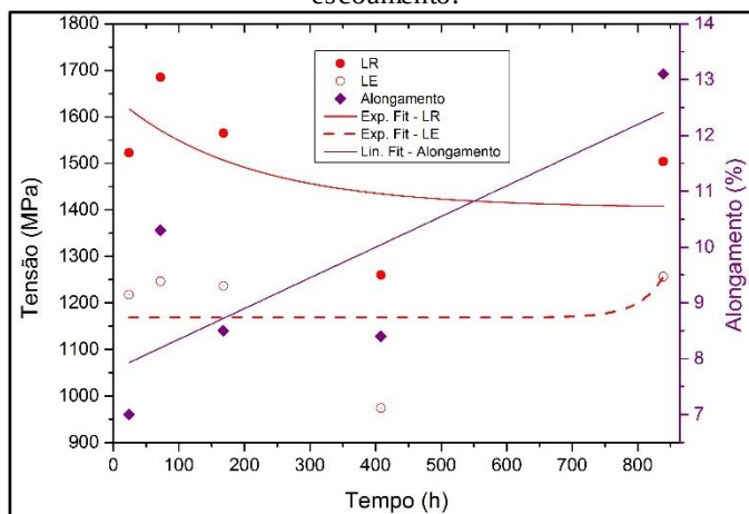
Figura 4.75 – Variação dos limites de resistência, limite de escoamento e alongamento em função do tempo de tratamento de austêmpera a 280°C para a liga 2 (1,94% Si). Legenda: LR – limite de resistência e LE – limite de escoamento.
