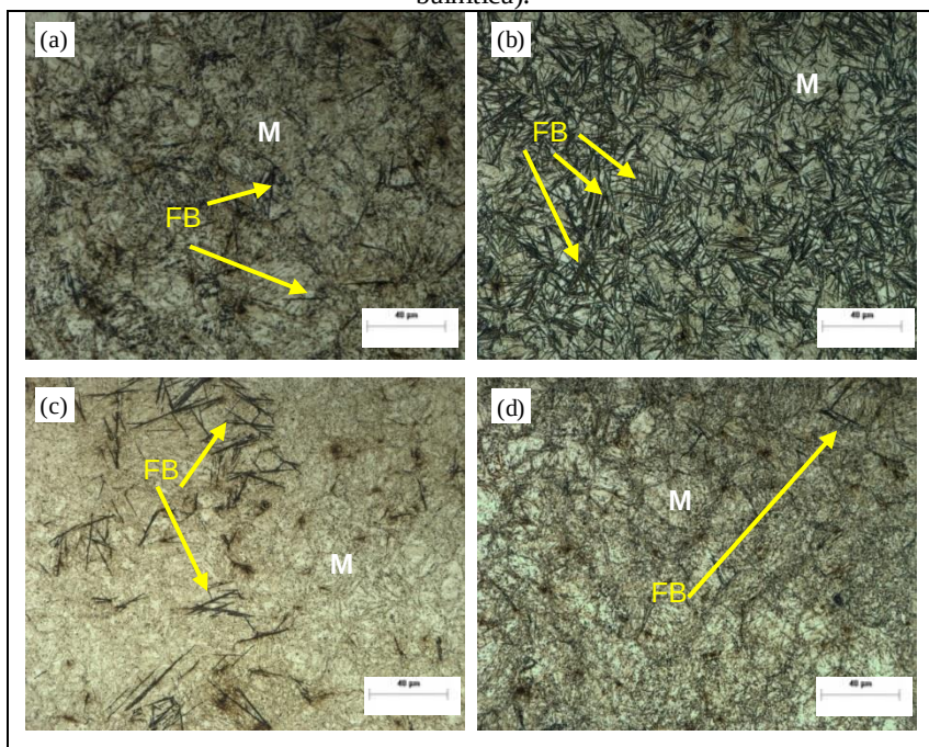
Figura 4.13 - Microestrutura das amostras austemperadas a 280^{\circ}C por 3 horas: (a) liga 1, (b) Liga 2, (c) Liga 3 e (d) Liga 4 . Microscopia óptica (MO). Ataque Le Pera. Aumento em função da escala. Legenda: M (martensita), FB (ferrita bainítica).
