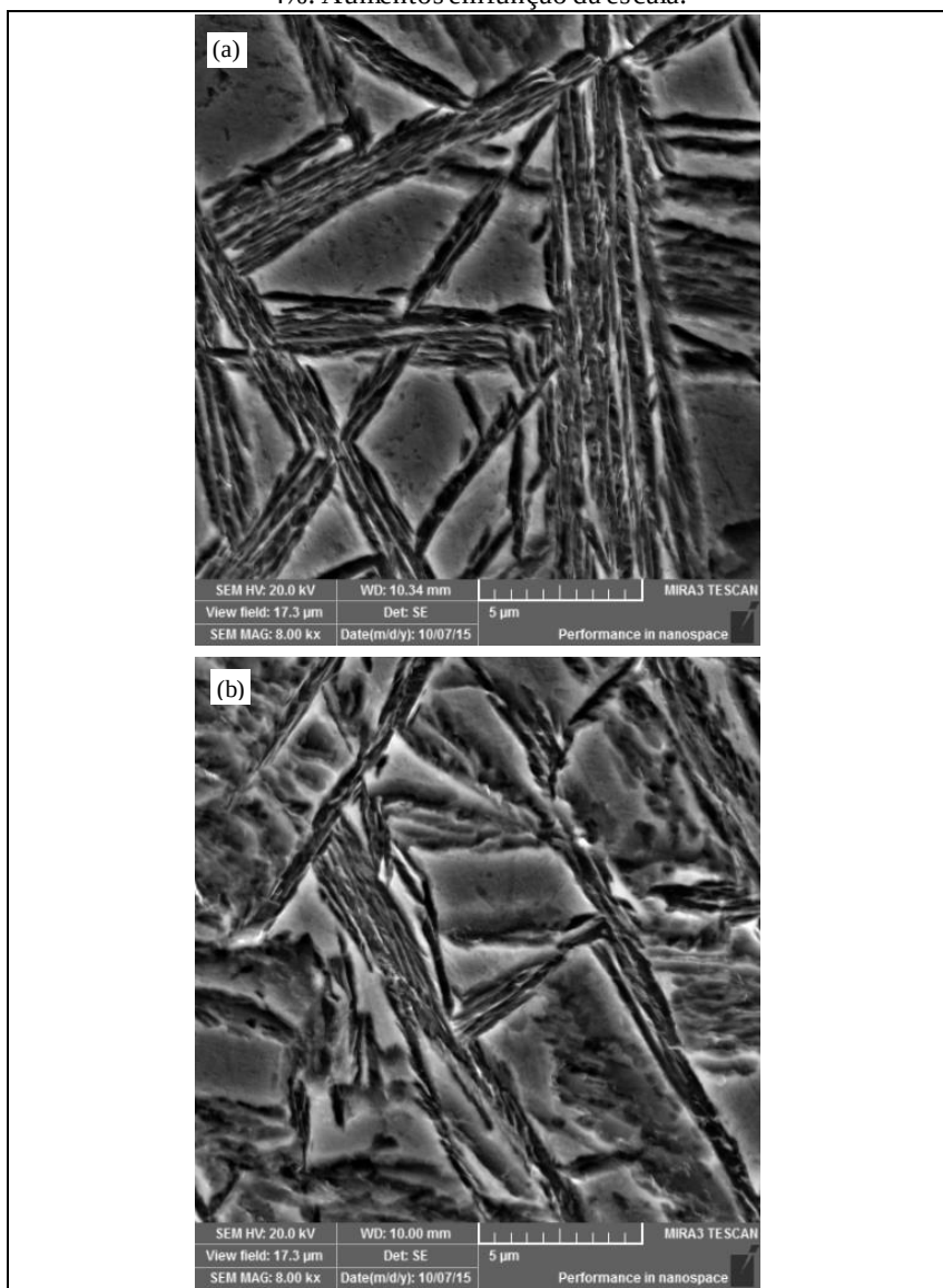
Figura 4.44 - Micrografias de amostras das Ligas 3 (a), Liga 4 (b), austenitizadas a 1150°C e austemperadas a 280°C por 12 horas. Reagente Picral 4%. Aumentos em função da escala.
