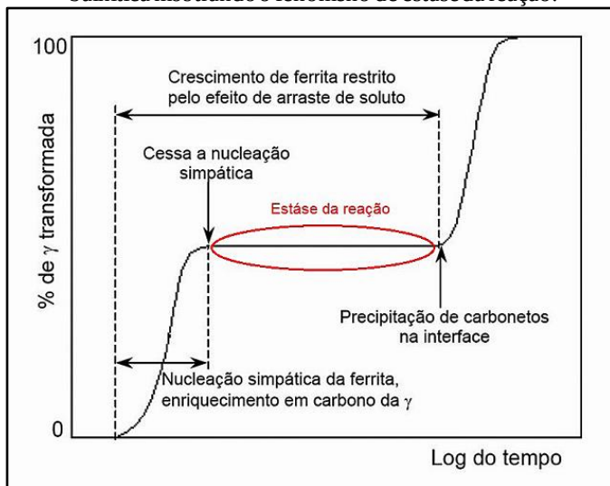
Figura 2.22 - Diagrama esquemático da cinética global da transformação bainítica mostrando o fenômeno de estase da reação.
