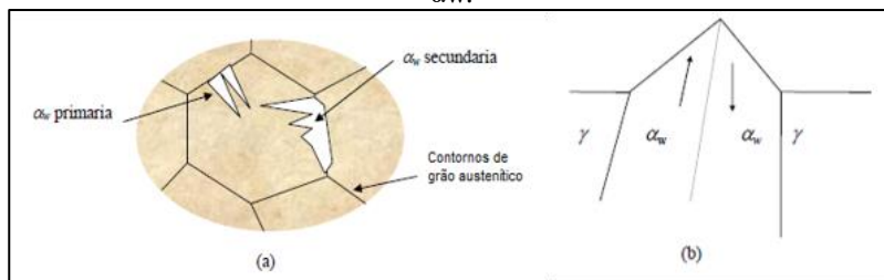
Figura 2.7 - Esquema que representa a morfologia da ferrita de Widmanstätten ( \alpha_w ). Sendo: (a) \alpha_w - primária e secundária e (b) arranjo mútuo de placas de \alpha_w .
