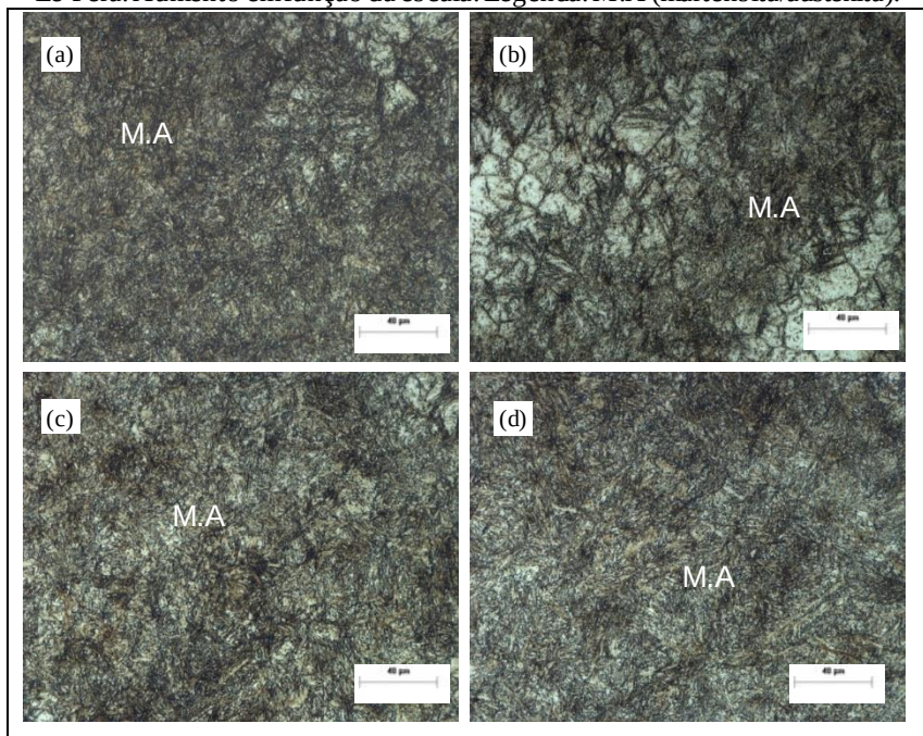
Figura 4.10 - Microestrutura das amostras austemperadas a 280°C por 1 hora: (a) liga 1, (b) Liga 2, (c) Liga 3 e (d) Liga 4. Microscopia óptica (MO). Ataque Le Pera. Aumento em função da escala. Legenda: M.A (martensita/austenita).
