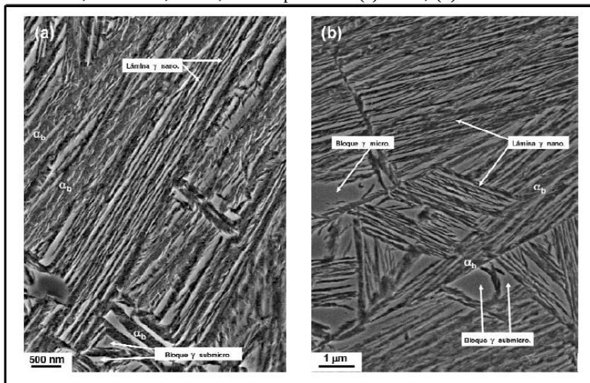
Figura 2.26 – Micrografias obtidas por MEV indicando a presença de ferrita bainítica, austenita em filmes (nanométricos) e em bloco (micro e submicrométrico) em amostras do aço 0,93%C – 2,9%Si – 0,77%Mn – 0,45%Cr – 0,16%Ni, austemperadas a: (a) 220°C; (b) 250°C.
