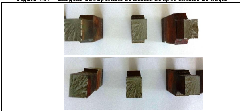
Figura 4.84 – Imagens da superfície de fratura de após ensaios de tração
