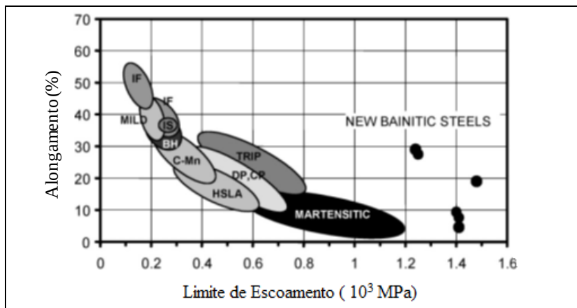
Figura 2.31- Comparação entre o limite de escoamento e alongamento dos novos aços bainíticos e outras classes de aços, incluindo: intersticial livre (IF); carbono-mangânês (CMN), bake hardenable (BH); dual phase (DP); complex phase (CP).
