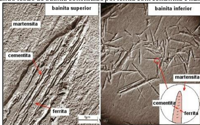
Figura 2.12 – Morfologia da ripa de ferrita bainítica da transformação de um aço de médio teor de carbono e silício. (a) Bainita Superior mostrando os feixes de bainita com cementita em uma matriz martensítica; (b) Bainita Inferior mostrando feixes de bainita constituído por ferrita com cementita e martensita.
