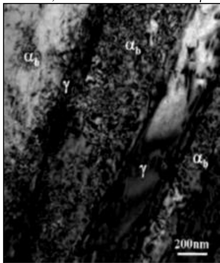
Figura 2.15 - Imagem de microscopia eletrônica de transmissão em campo claro mostrando emaranhados de discordâncias na interface ferrita/austenita na microestrutura bainítica, onde: \alpha_b é ferrita bainítica e \gamma é austenita retida.
