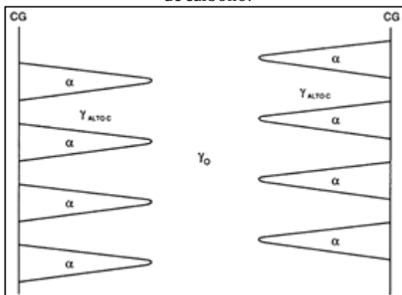
Figura 2.21 - Representação do crescimento da ferrita bainítica ( \alpha ), a partir do contorno de grão da austenita (CG, \gamma_0 ), criando zonas de austenita com alto teor de carbono.
