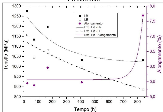
Figura 4.74 – Variação dos limites de resistência, limite de escoamento e alongamento em função do tempo de tratamento de austêmpera a 280°C para a liga 1 (liga base). Legenda: LR – limite de resistência e LE – limite de escoamento.
