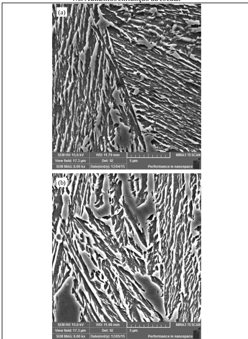
Figura 4.47 - Micrografias de amostras das Ligas 1 (a), Liga 2 (b), austenitizadas a 1150°C e austemperadas a 370°C por 12 horas. Reagente Picral 4%. Aumentos em função da escala.
