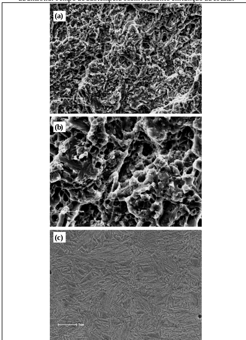
Figura 4.90 – Imagens das superfícies de fratura e microestrutura das amostras ensaiadas para a liga 2. Sendo: (a) e (b) superfície de fratura e (c) microestrutura da amostra. Tempo de austêmpera 168h. Aumento em função da escala.
