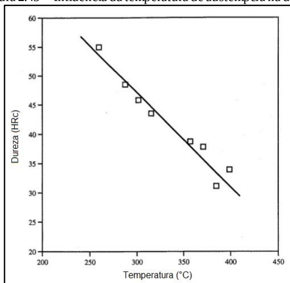
Figura 2.45 – Influência da temperatura de austêmpera na dureza
