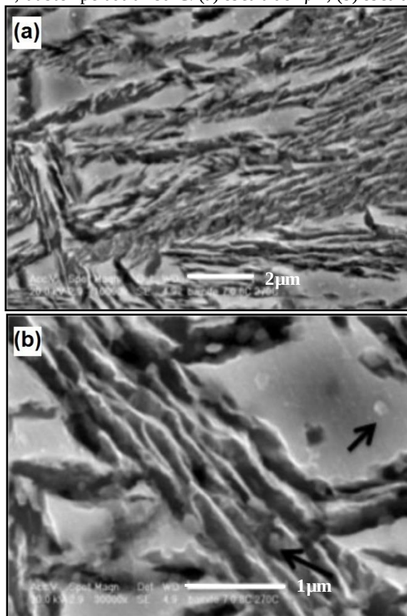
Figura 2.27 – Micrografias obtidas por MEV indicando a presença de austenita em filmes e em bloco em uma amostra de aço 0,73%C – 1,82%Si – 1,47%Cr – 4,12%Ni, austemperada a 280°C: (a) escala de 2µm; (b) escala de 1µm.
