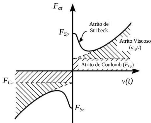
Figura 4.8 – Curva estática da força de atrito e suas principais componentes.
