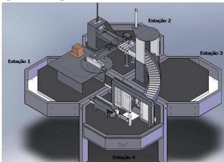
Figura 3.2 – Visão geral da bancada SPCS.
