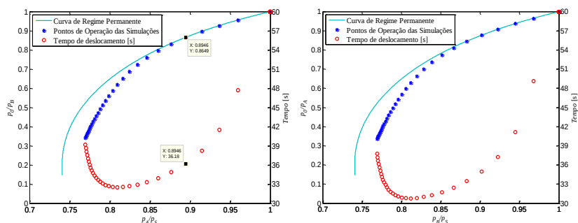
Figura 5.5 - Relação do tempo de deslocamento com o ponto de operação para avanço (esquerda) e retorno (direita).
