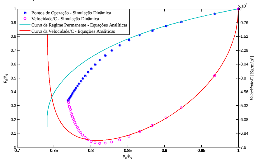
Figura 6.4 - Comparação das equações analíticas com os dados da simulação dinâmica para o movimento de retorno.
