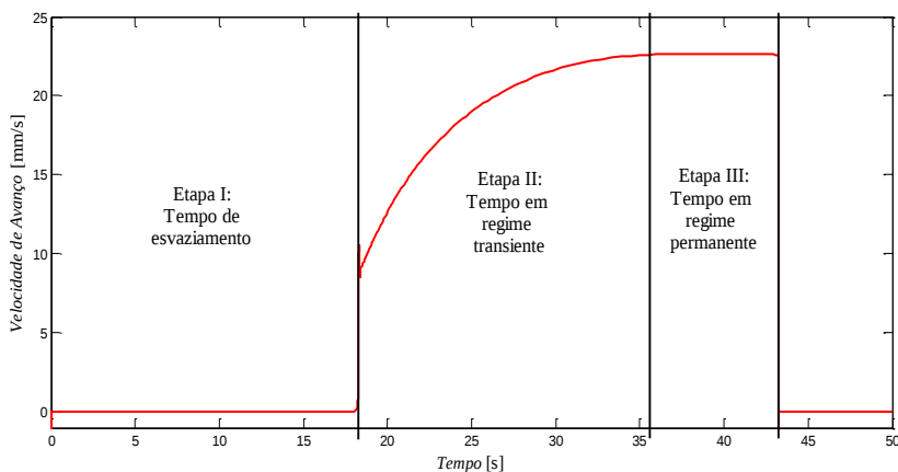
Figura 5.11 - Principais etapas do movimento de deslocamento.
