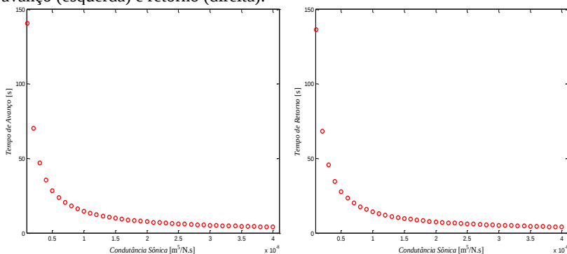
Figura 5.9 – Relação de tamanho de válvula com tempo de deslocamento para avanço (esquerda) e retorno (direita).
