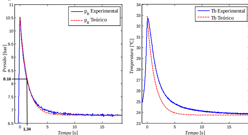
Figura 4.4 – Curvas resultantes da troca de calor entre o atuador e o ambiente.
