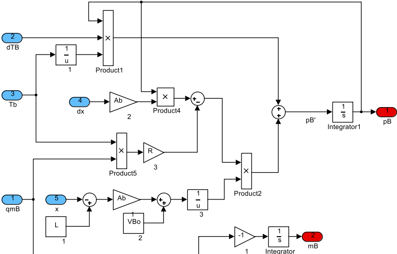
Figura D.3 – Diagrama de blocos da equação da continuidade da câmara B.
