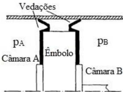
Figura 4.6 – Representação das vedações no êmbolo.
