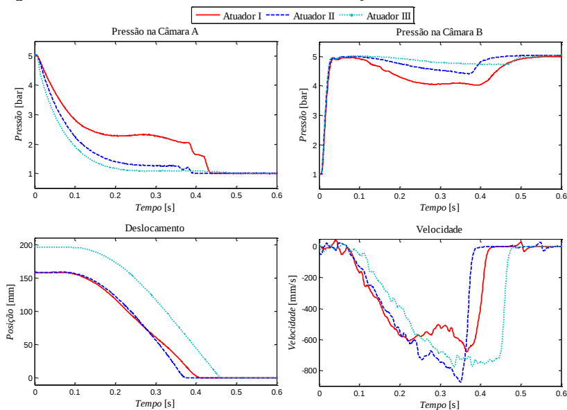
Figura 6.6 – Variáveis de estado observadas nos experimentos.
