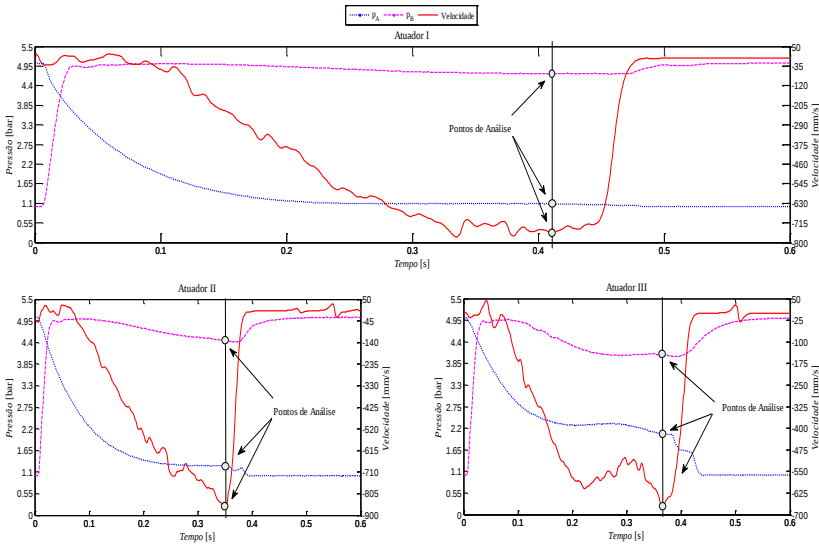
Figura 6.8 – Pontos de análise dos resultados experimentais.
