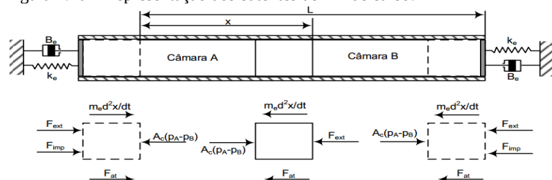
Figura 4.10 – Representação dos batentes de fim de curso.
