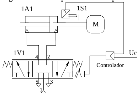
Figura 2.6 – Exemplo de um servoposicionador pneumático.
