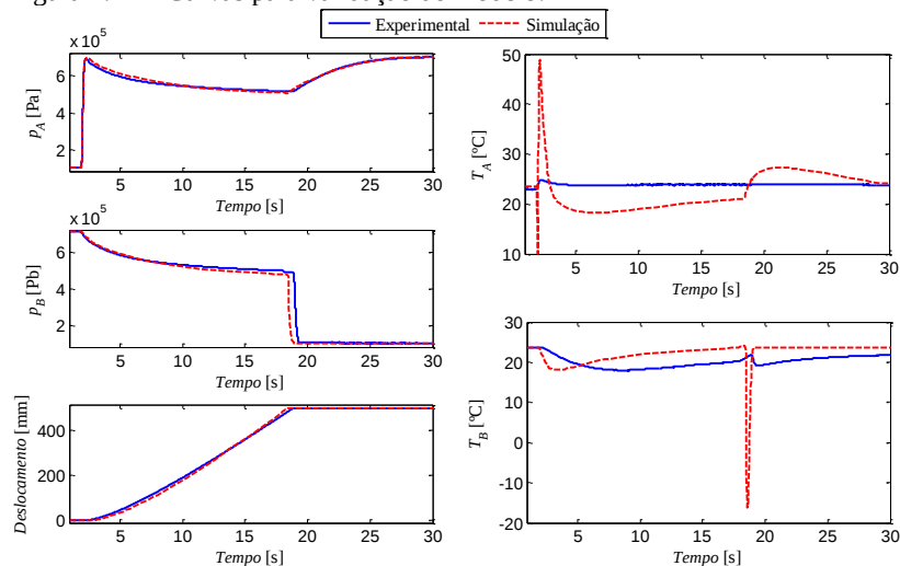
Figura 4.11 – Curvas para validação do modelo.
