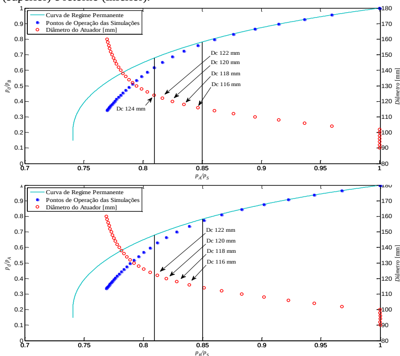
Figura 5.8 – Delimitação dos pontos ótimos de operação para o avanço (superior) e retorno (inferior).
