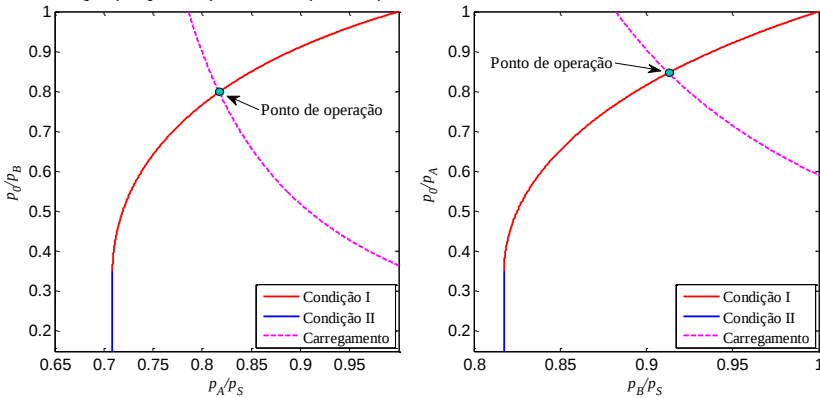
Figura 5.2 – Curvas de regime permanente e de carregamento para o movimento de avanço (esquerda) e recuo (direita).
