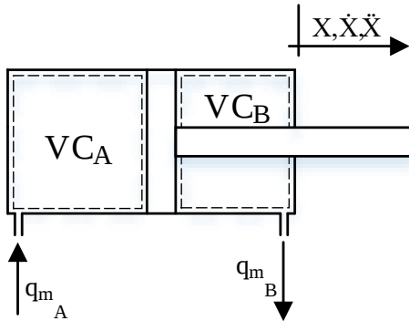
Figura 4.5 – Volumes de controle de um atuador pneumático.
