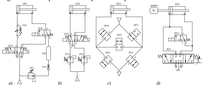
Figura 2.8 – Exemplos de circuitos pneumáticos para aumento de eficiência.
