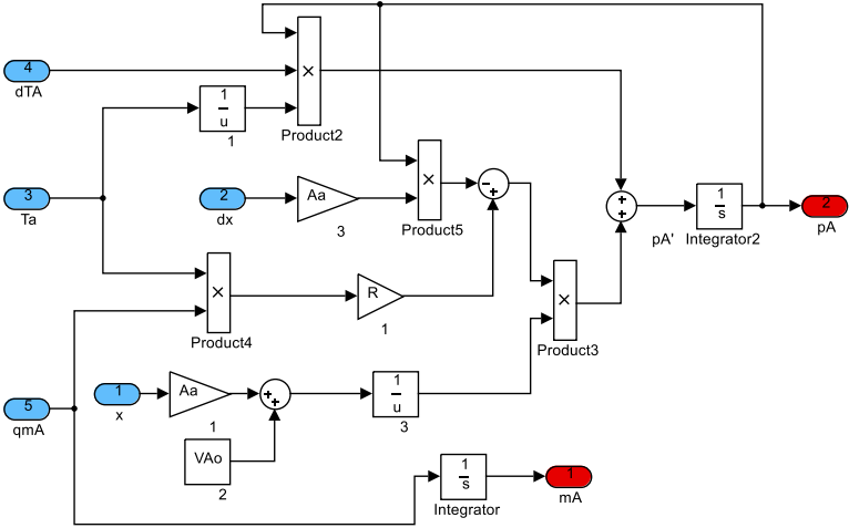
Figura D.2 – Diagrama de blocos da equação da continuidade da câmara A.
