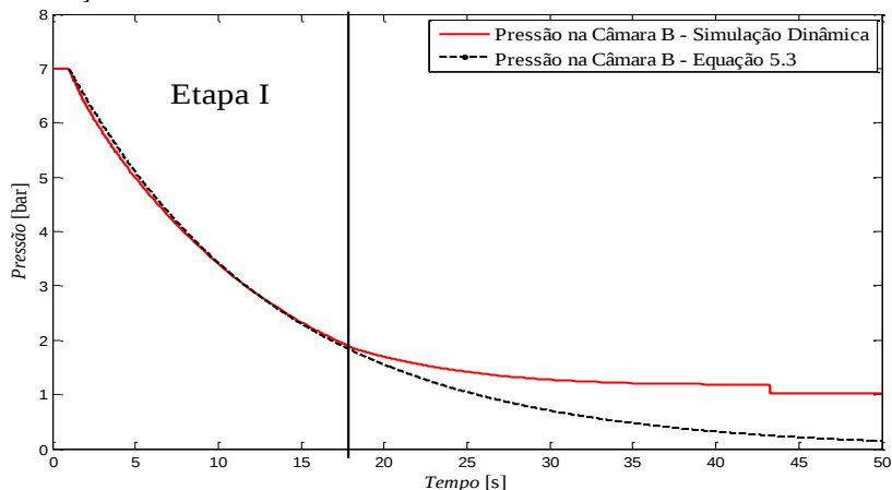
Figura 5.13 – Comparação dos resultados obtidos com a Equação (5.3) e com a simulação dinâmica
