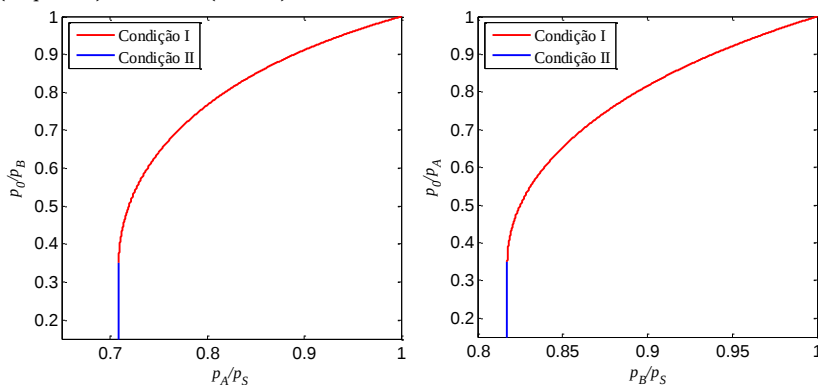
Figura 5.1 – Curvas de regime permanente para o movimento de avanço (esquerda) e retorno (direita).
