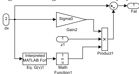
Figura D.6 – Diagrama de blocos da equação G(v) do modelo de atrito.
