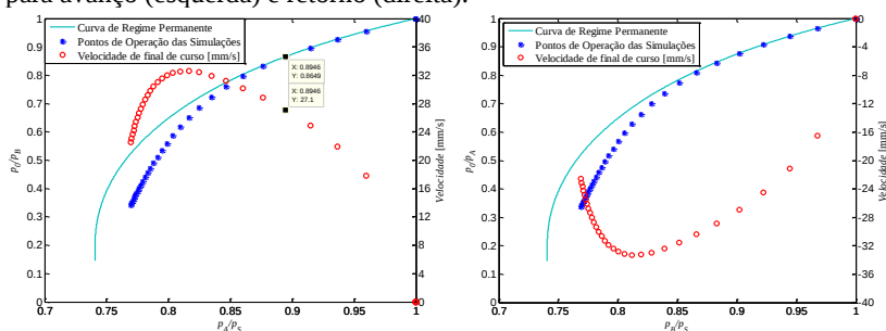
Figura 5.6 - Relação de velocidade de fim de curso com o ponto de operação para avanço (esquerda) e retorno (direita).
