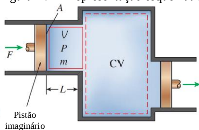
Figura B.2 – Representação esquemática do trabalho de escoamento
