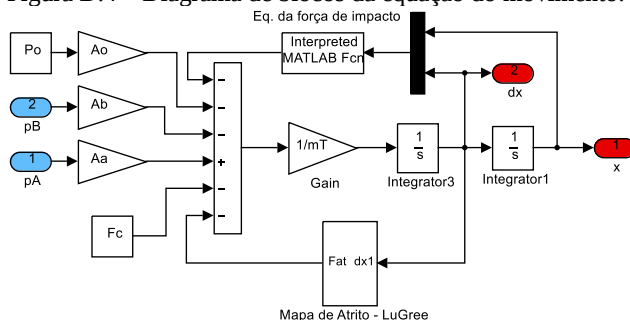
Figura D.4 – Diagrama de blocos da equação do movimento.
