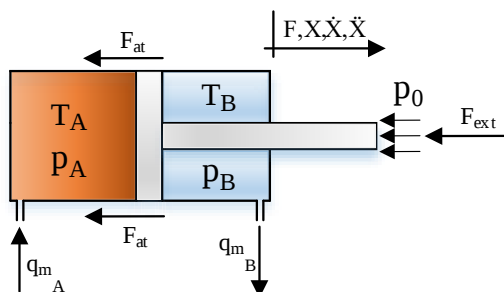
Figura 4.2 - Principais variáveis e forças que atuam em um cilindro pneumático.
