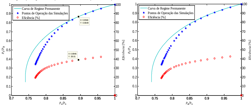
Figura 5.7 – Relação da eficiência energética com o ponto de operação para avanço (esquerda) e retorno (direita).
