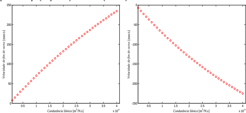
Figura 5.10 - Relação de tamanho de válvula com velocidade de fim de curso para avanço (esquerda) e retorno (direita).
