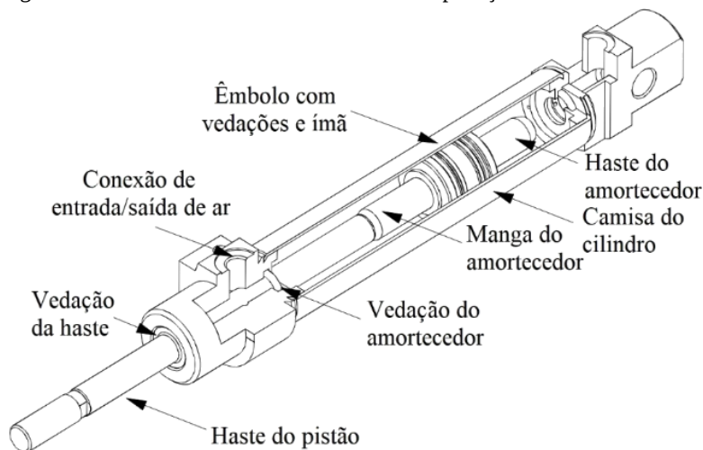
Figura 2.2 – Vista em corte de um atuador de dupla ação.
