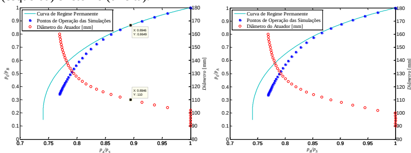
Figura 5.4 – Relação do diâmetro com o ponto de operação para avanço (esquerda) e retorno (direita).
