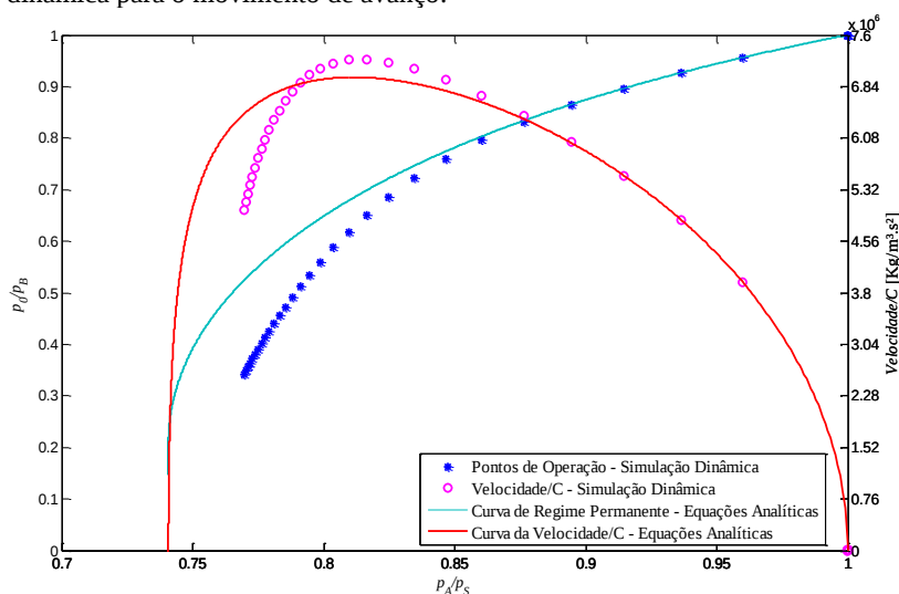
Figura 6.2 – Comparação das equações analíticas com os dados da simulação dinâmica para o movimento de avanço.
