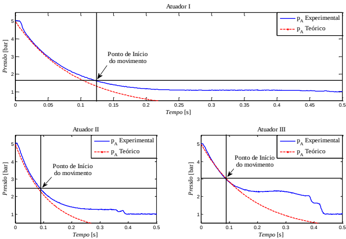
Figura 6.7 – Comparação da pressão teórica e experimental da câmara A de cada atuador.
