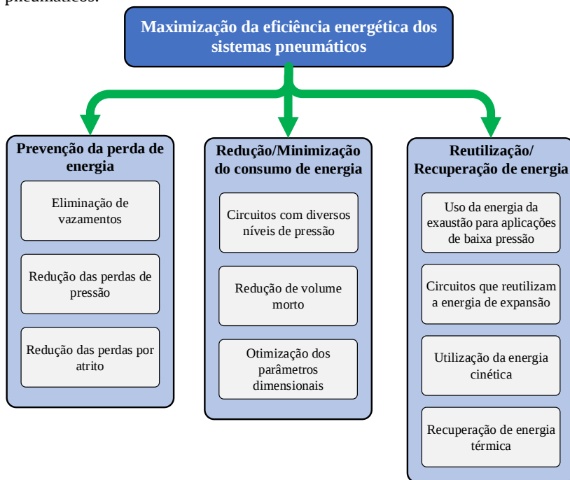
Figura 2.7 – Estratégias para maximização da eficiência energética dos sistemas pneumáticos.
