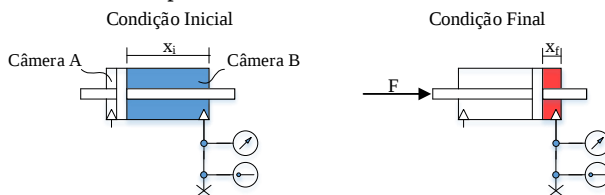
Figura 4.3– Diagrama esquemático do experimento para determinação da constante de tempo.
