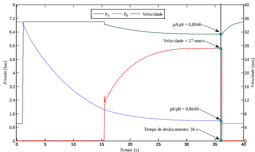
Figura 5.3 – Simulação dinâmica para um atuador de 110 mm
