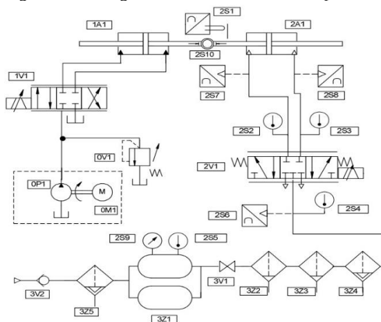
Figura 3.3 – Diagrama do circuito hidráulico-pneumático da bancada IBYTU
