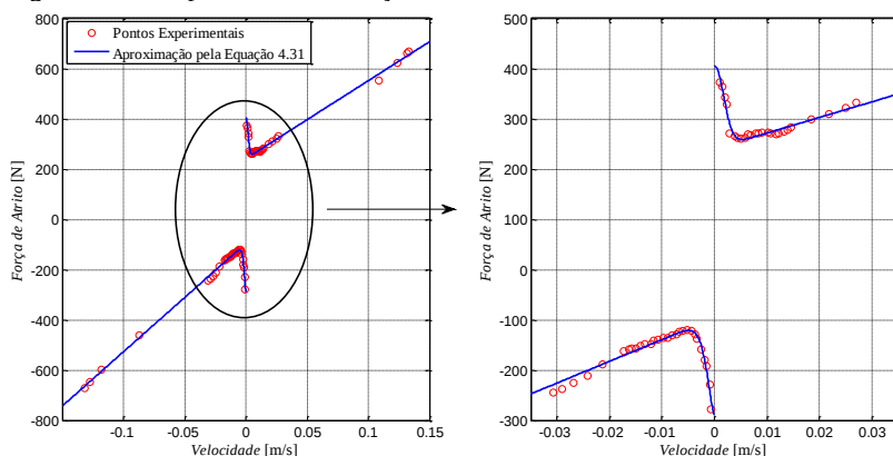
Figura 4.9 – Mapa estático da força de atrito.
