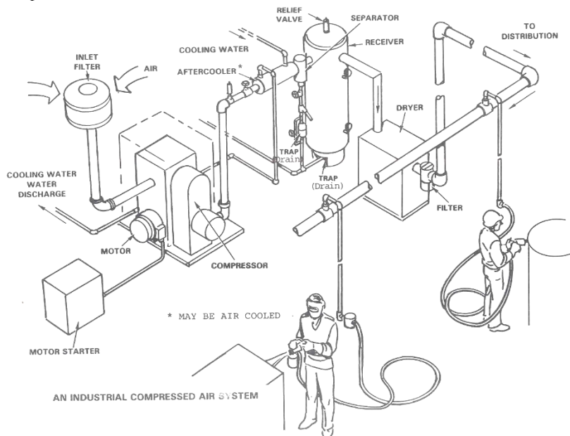
Figura 2.1 – Sistema de produção, condicionamento e distribuição de ar comprimido.
