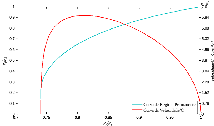
Figura 6.1 – Análise da velocidade de avanço em regime permanente
