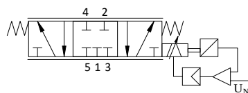
Figura 2.4 – Simbologia de uma válvula de controle direcional proporcional.
