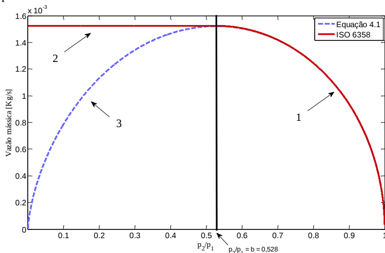
Figura 4.1 – Vazão mássica através de uma válvula em função da razão de pressões.
