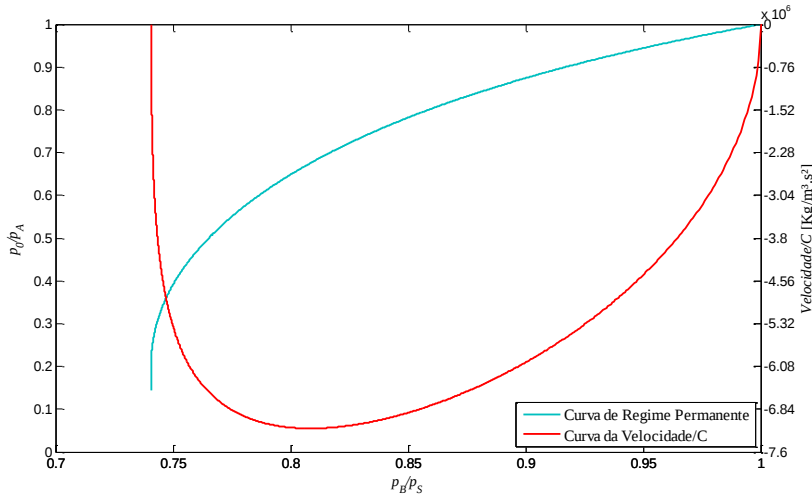
Figura 6.3 - Análise da velocidade de retorno em regime permanente.
