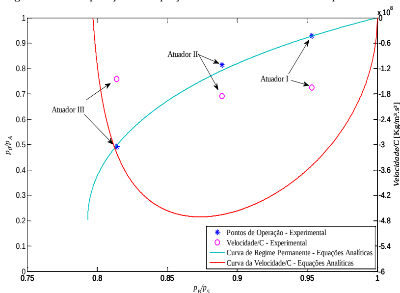
Figura 6.9 - Comparação das equações analíticas com os dados experimentais.
