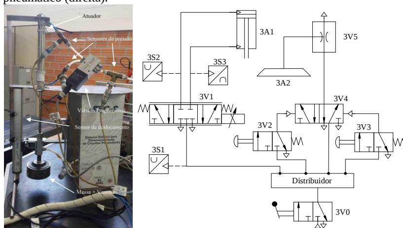
Figura 3.6 - Estação 3 da bancada SPCS (esquerda) e diagrama do circuito pneumático (direita).
