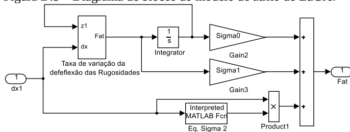
Figura D.5 – Diagrama de blocos do modelo de atrito de LuGre.
