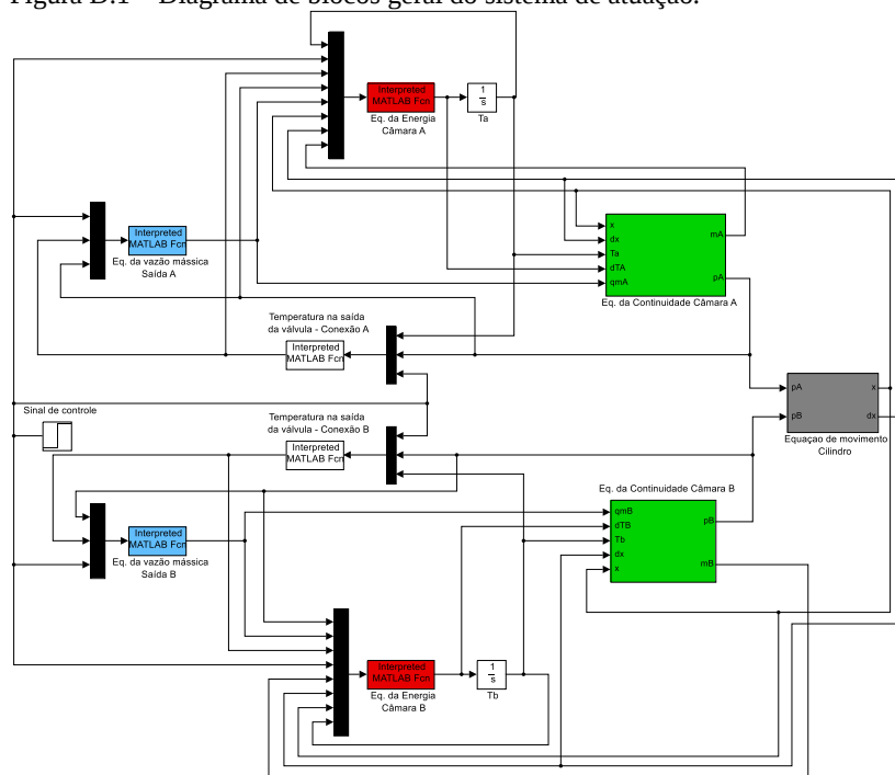
Figura D.1 – Diagrama de blocos geral do sistema de atuação.
