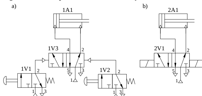
Figura 2.5 - Exemplos de sistemas de atuação discretos.
