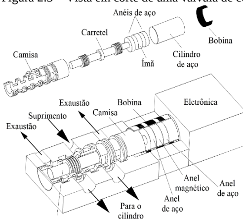
Figura 2.3 – Vista em corte de uma válvula de controle direcional proporcional.
