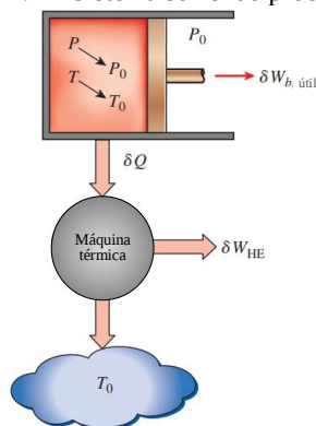
Figura B.1 – Sistema sofrendo processo reversível
