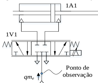
Figura 4.12 – Ponto de observação para o cálculo da exergia.
