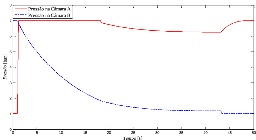
Figura 5.12 – Comportamento das pressões durante o deslocamento do atuador
