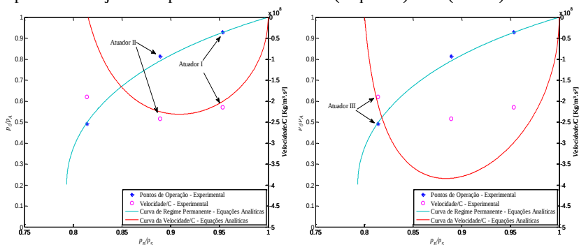
Figura 6.10 – Comparação das equações analíticas com os dados experimentais e parâmetros ajustados para os atuadores I e II (esquerda) e III (direita).
