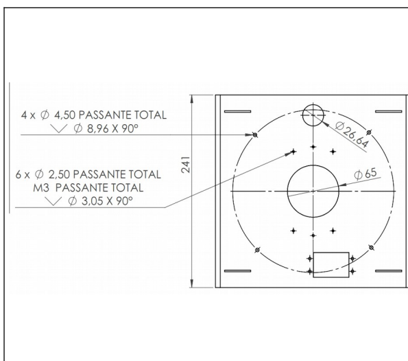
Tambor montado (destaque disco inferior)
