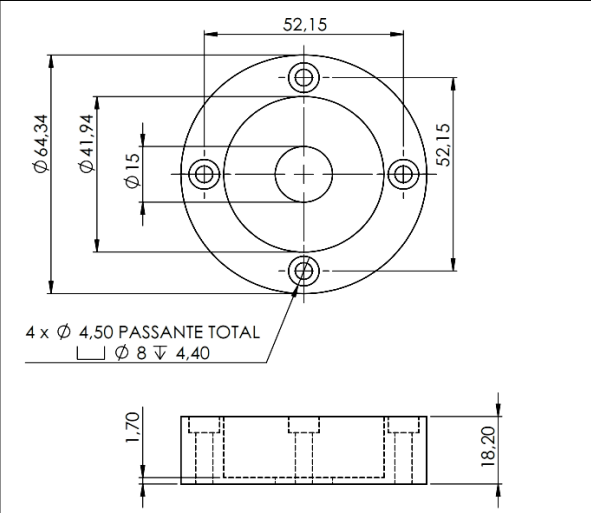
Caixa Carrossel (vista lateral)
