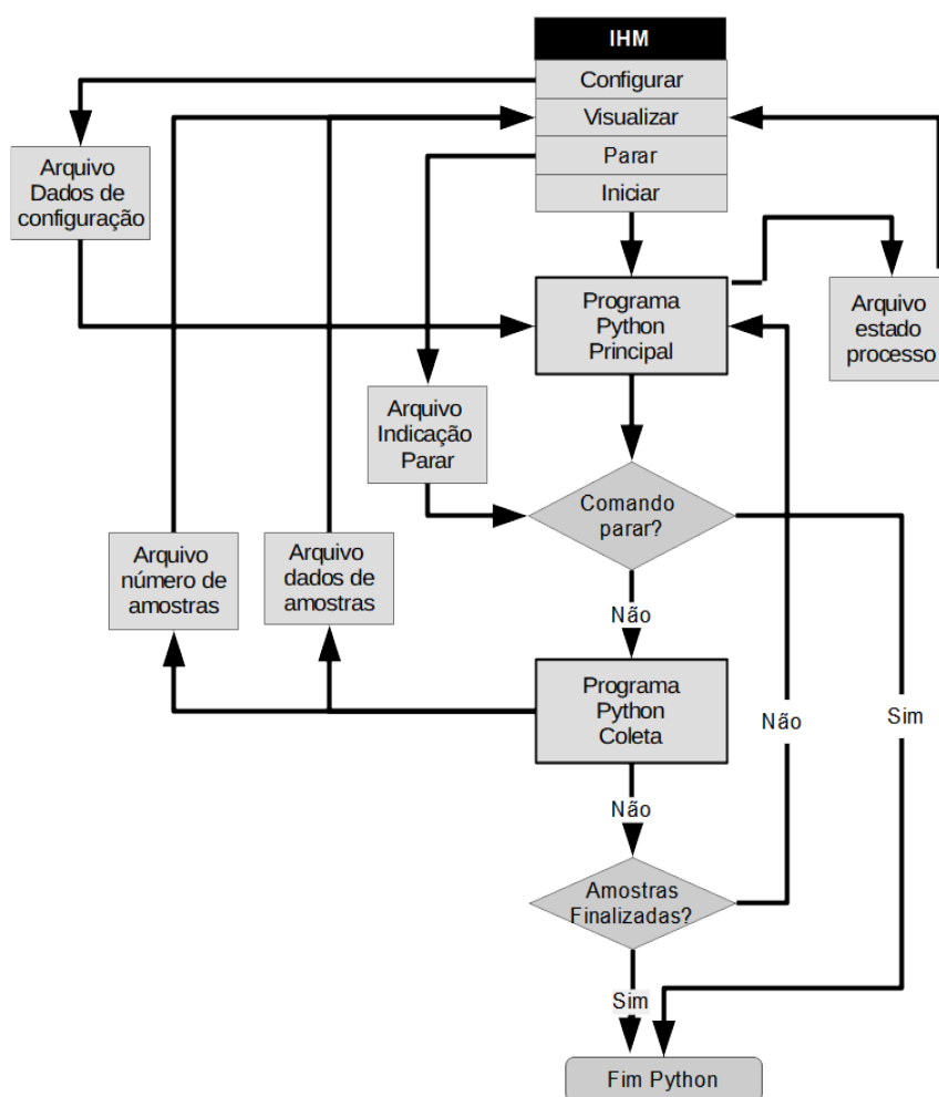
FIGURA 31 - Fluxograma simplificado do acionamento via IHM.
