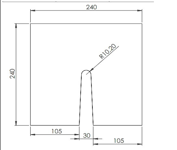
Caixa Carrossel (vista superior)
