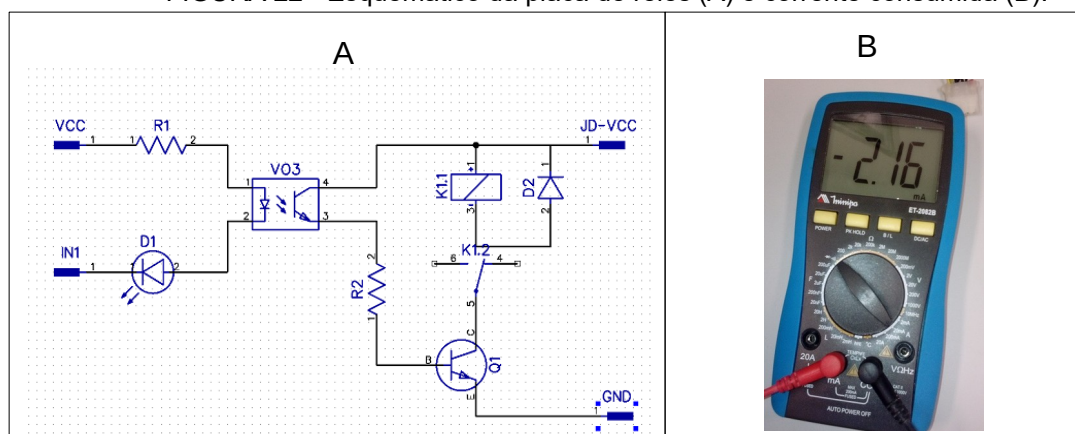
FIGURA 22 - Esquemático da placa de relés (A) e corrente consumida (B).
