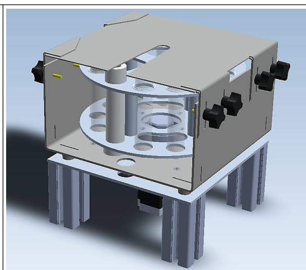
Montagem base do carrossel
