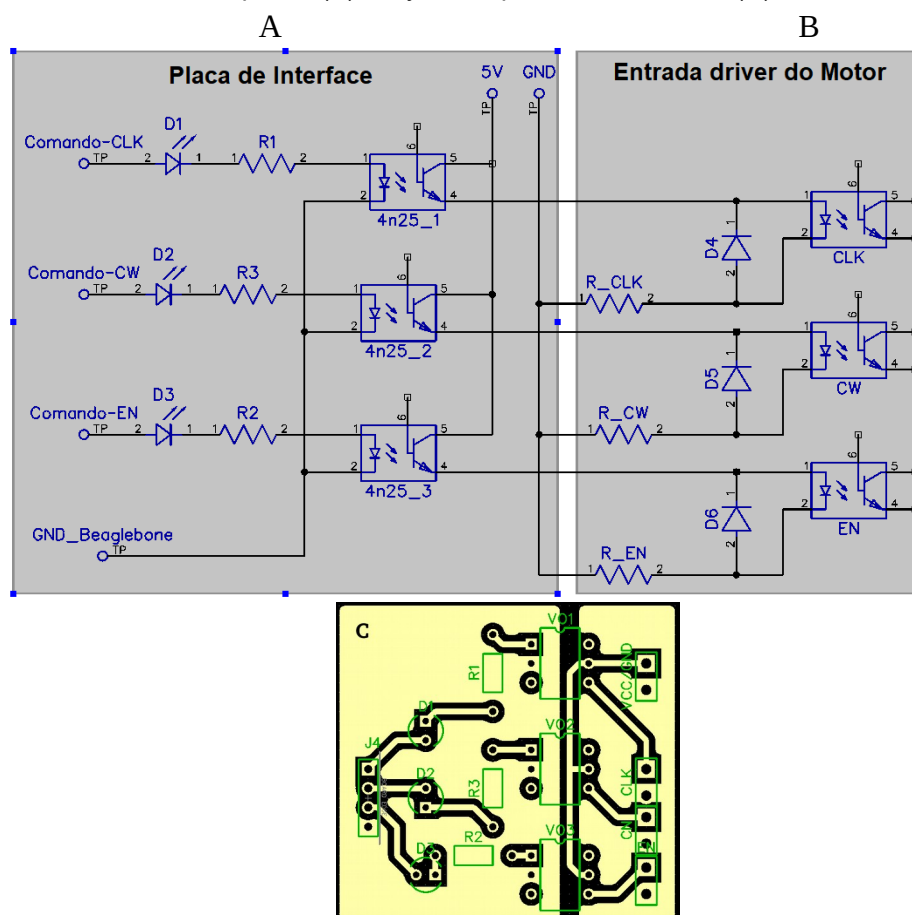
FIGURA 25 - Esquemático da placa de interface (A), esquemático entrada do driver do motor de passo (B) e layout da placa desenvolvida (C).
