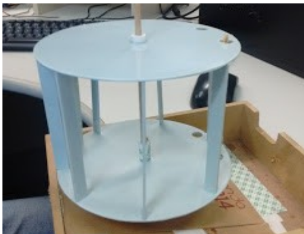
FIGURA 10 - Primeira concepção de carrossel testada
