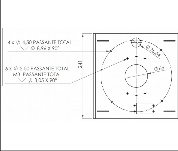
Caixa Carrossel (vista frontal)
