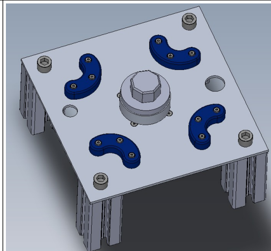
Montagem base do carrossel
