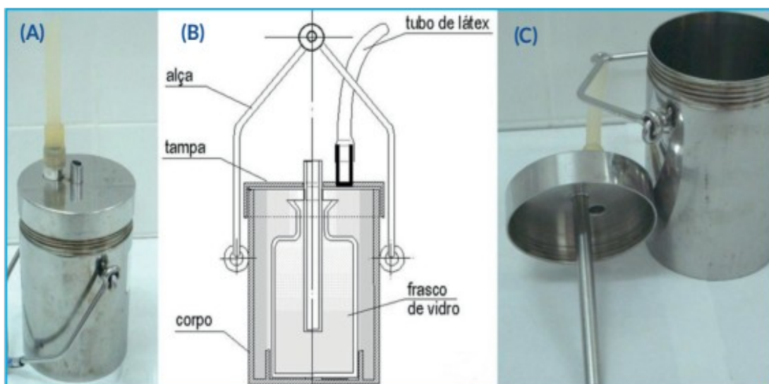
FIGURA 2 - Batiscafo. (A) fechado. (B) ilustração em corte. (C) Aberto.
