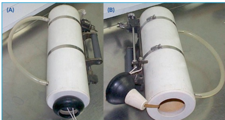
FIGURA 3 - Garrafa de Van Dorn de fluxo vertical. (A) Garrafa fechada. (B) Garrafa aberta e pronta para uso.
