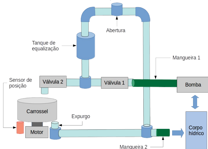
FIGURA 12 - Componentes módulo mecânico.
