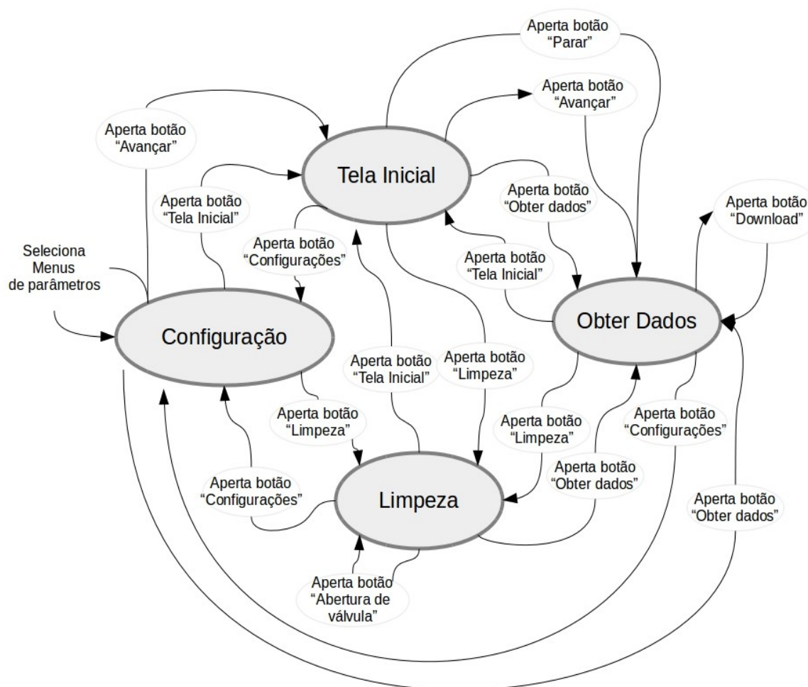
FIGURA 15 - Diagrama de modos da Interface Humano-Máquina.
