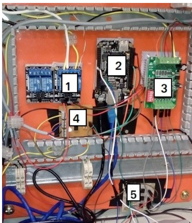
FIGURA 26 - Painel elétrico construído.
