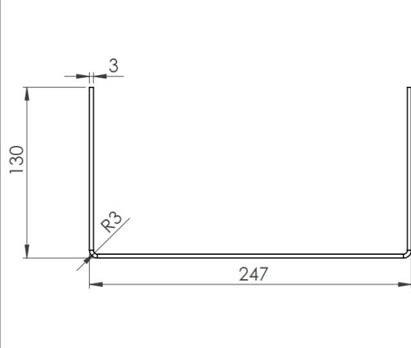
Trava de tampa do carrossel
