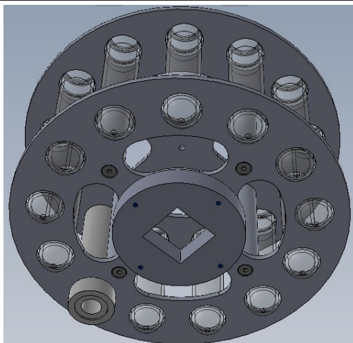
Tambor montado (destaque disco inferior)
